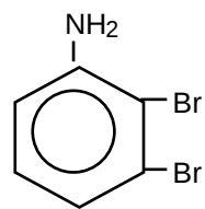
2,3-dibromoaniline
